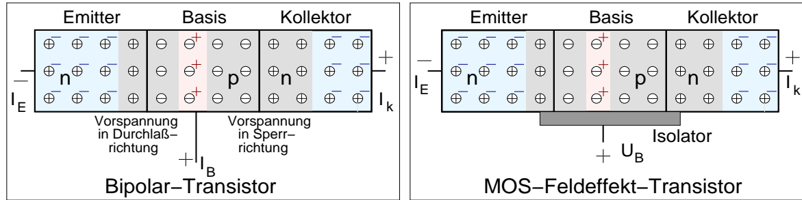
Grundtypen von Transistoren
