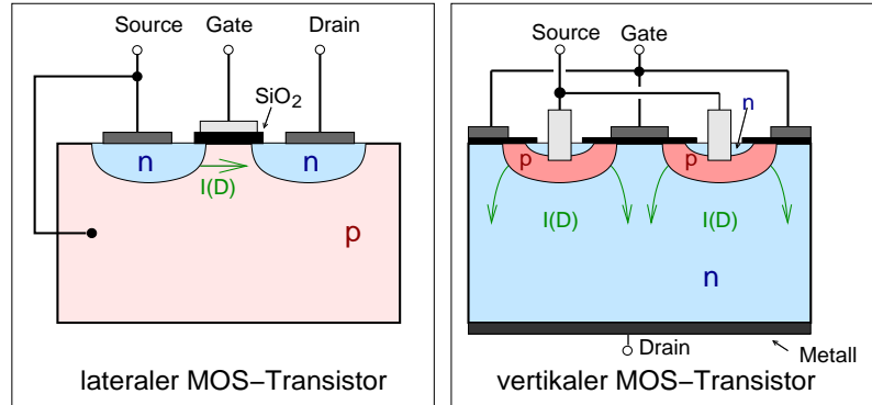
Bauarten von MOS-Feldeffekttransistoren
