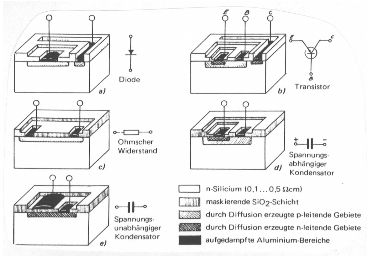
Halbleiter-Schaltungselemente
