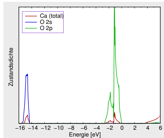
CaO (Ionenkristall)
