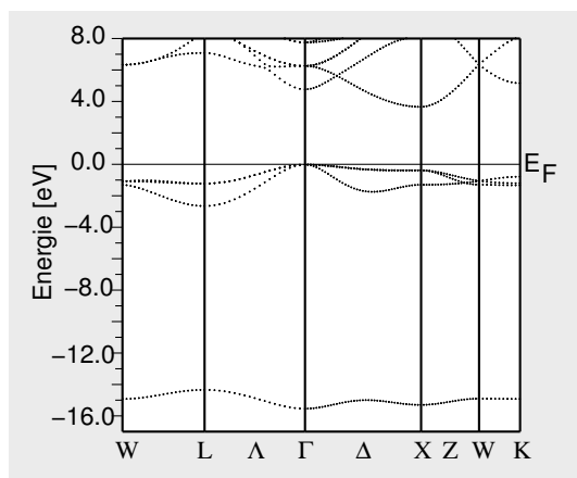
CaO (Ionenkristall)
