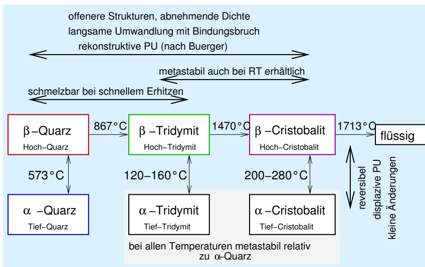
thermodynamisch stabile Normaldruckphasen
