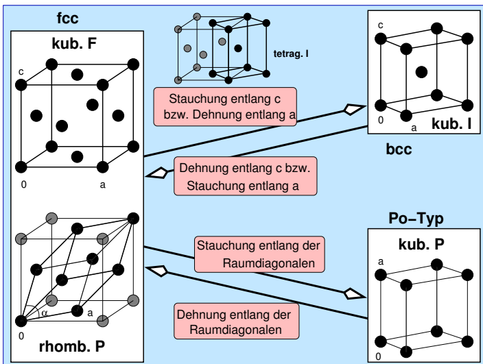
Verzerrungen von Metallpackungen
