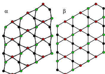
alpha- (RG P3 1 21) und beta- (RG P6 2 22) Quarz (nur Si-Positionen)
