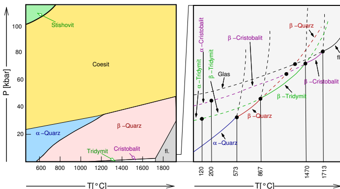
Phasenbeziehungen zwischen den verschiedenen SiO 2 -Modifikationen
