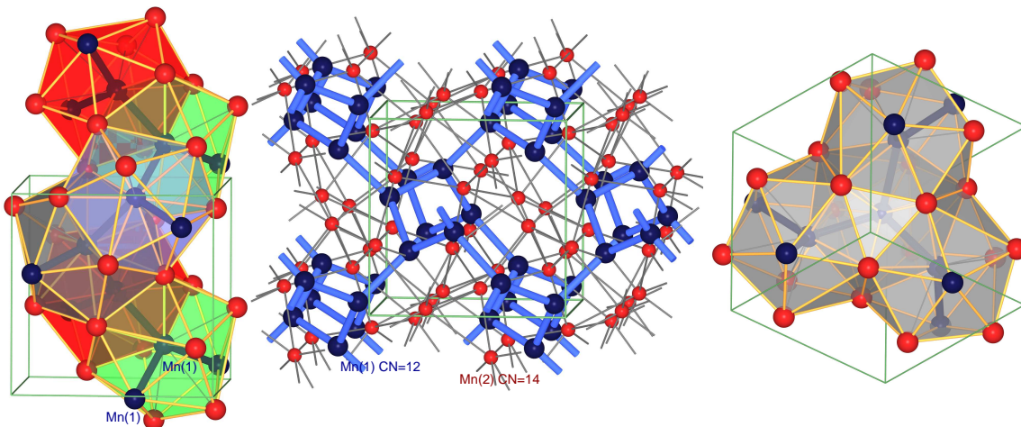
Kristallstruktur von \beta -Mangan ( oP20 , Raumgruppe P4_132 )
