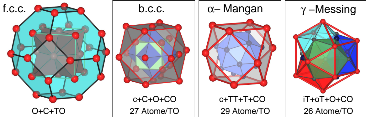
Parkettierungen des Raums mit gekappten Oktaedern (TO): f.c.c., b.c.c., \alpha -Mn, \gamma -Messing)
