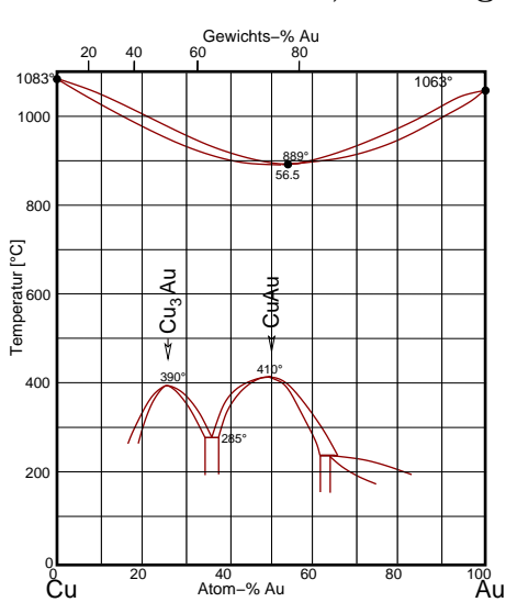
Phasendiagramm Cu-Au
