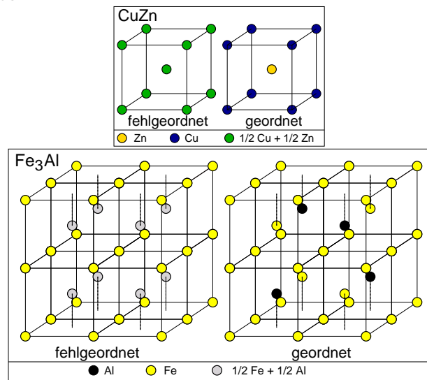
ausgeordnete b.c.c.-Strukturen: \beta -Messing und Fe 3 Al
