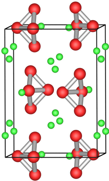
\text{Ba}_3\text{Si}_4
