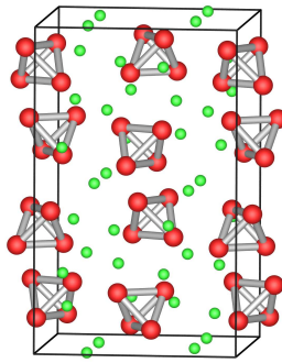
\text{KSn}
