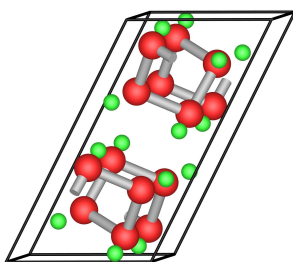
\text{LiAs}
