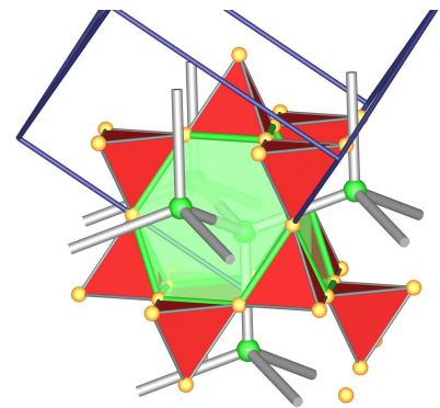
Mg-Umgebung: CN 12+4 (FK 16)
