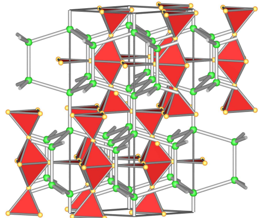
MgNi 2
