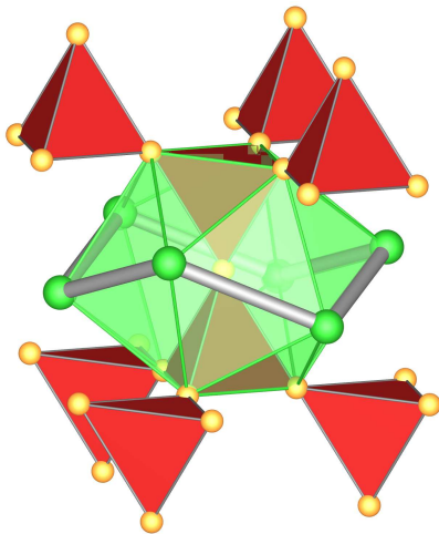
Cu-Umgebung: CN 6+6 (FK 12)
