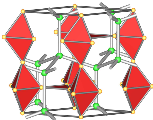
MgZn 2
