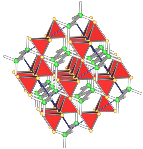
MgCu 2 : Gesamtstruktur
