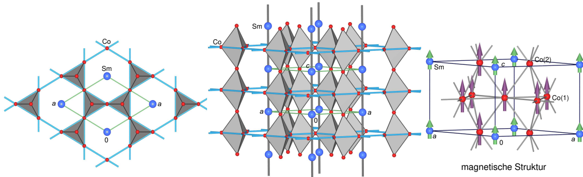
Kristallstruktur von SmCo 5 (CaCu 5 -Typ)
