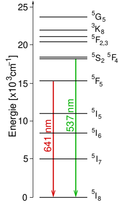
Termschema von Ho 3+
