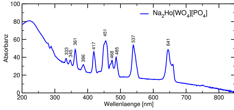
UV/VIS-Spektrum von Na 2 Ho[WO 4 ][PO 4 ]
