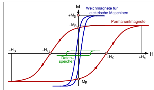
Hysteresekurven (nach Anwendungsbereich)
