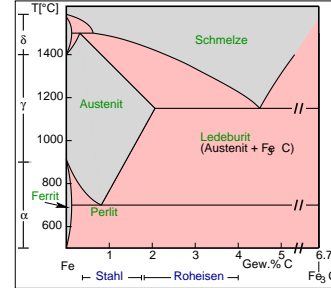
Phasendiagramm Fe-C
