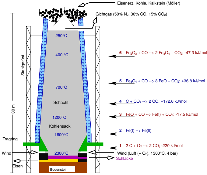
Hochofen (schematisch)
