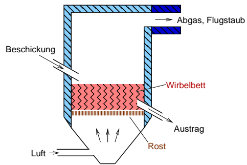
Wirbelschichtreaktor (schematisch)
