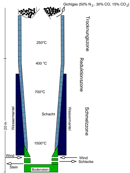
Wassermantelofen
