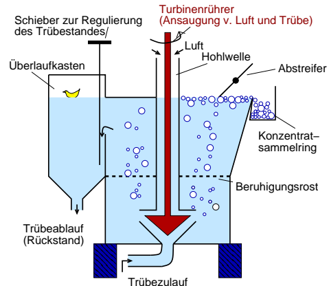
Flotationszelle
