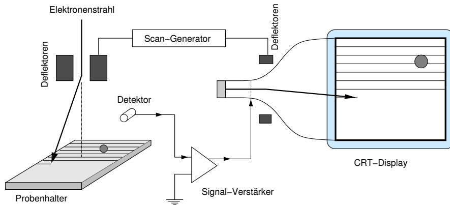
Funktionsprinzip des Rasterelektronenmikroskops
