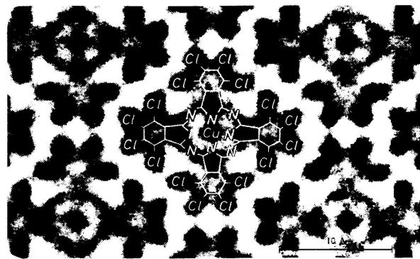
Durchstrahlungsaufnahme von chloriertem Kupferphthalocyanin (500 kV, Aufnahme \perp c-Achse )
