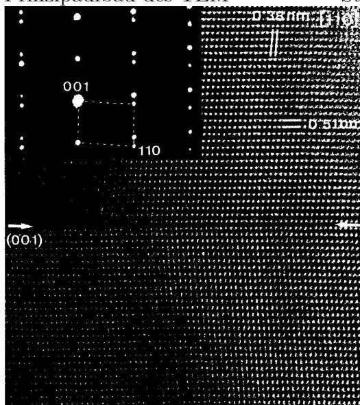
TEM-Aufnahme einer Zwillings ebene (entlang (001)) in YTaO_4 (links oben: Beugungsmuster)
