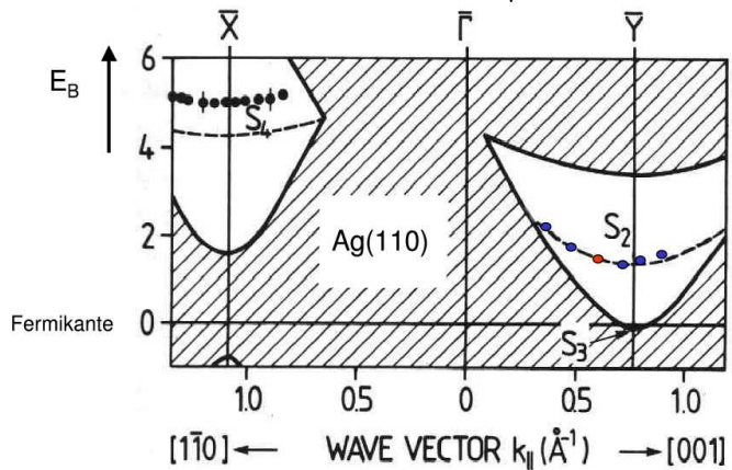
Meßpunkte in der Oberflächenbandstruktur
