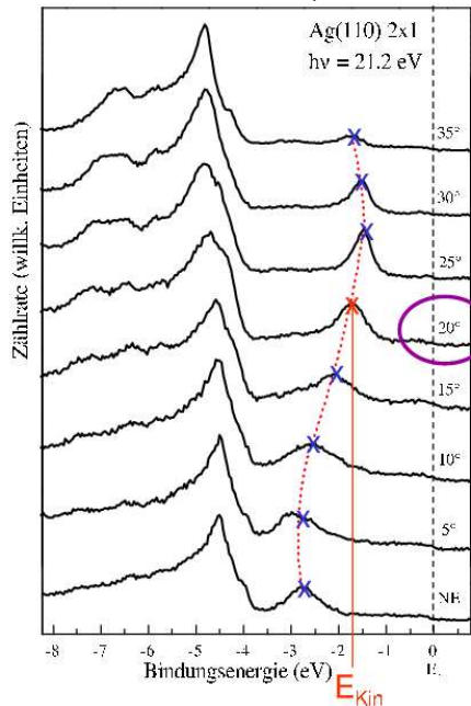
EDC-ARUPS-Spektren einer Ag(110)-Oberfläche
