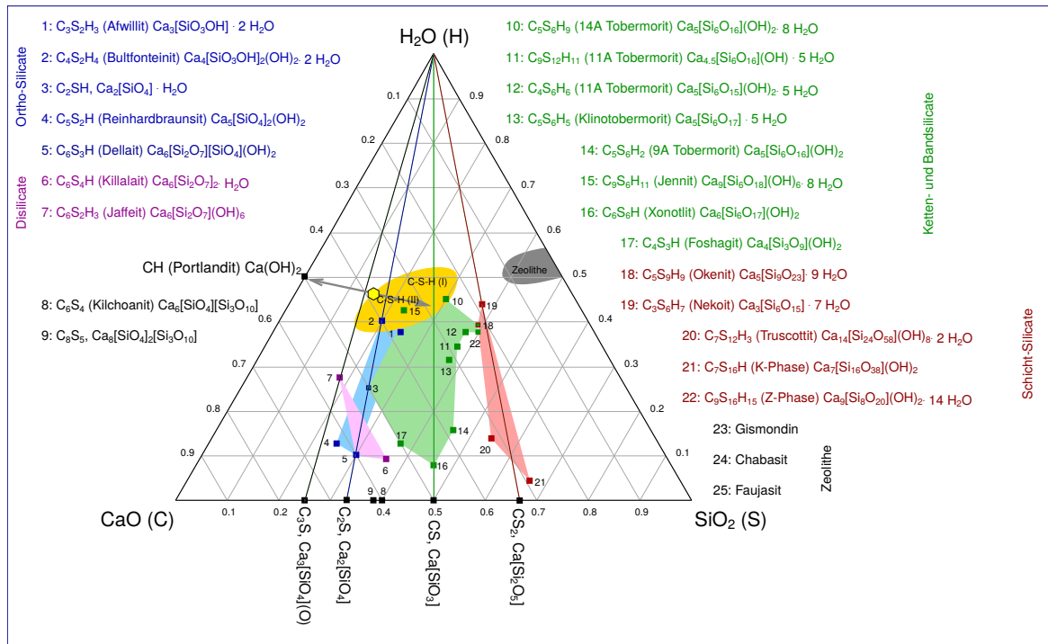
Übersicht: Kristalline CSH-Phasen
