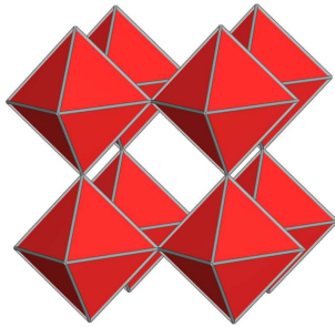
ReO 3 -Typ
