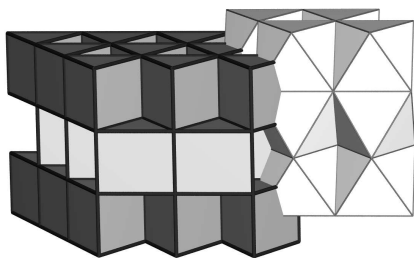
NiAs-Typ
