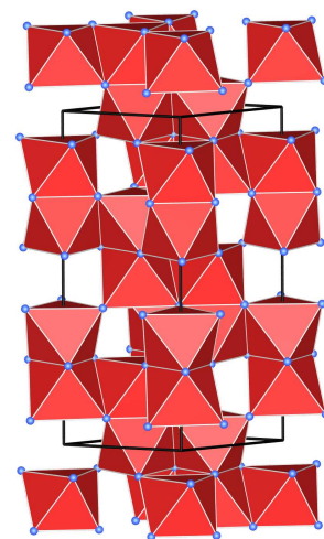
Korund-Struktur
