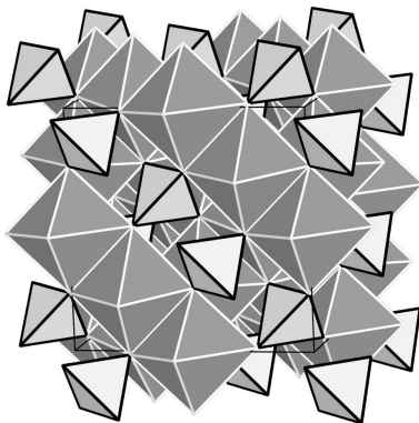
Spinell-Struktur)
