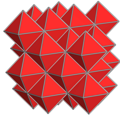
NaCl
