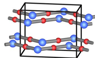
HgO: (rot)
