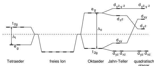
LFSE verschiedener 3d-Kationen in Oxiden
