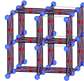
PtO:
