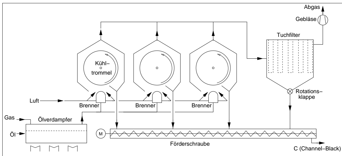
Channelblack-Verfahren (Degussa)
