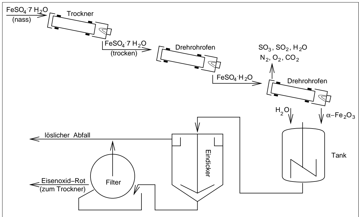
Herstellung von Copperas-Rot
