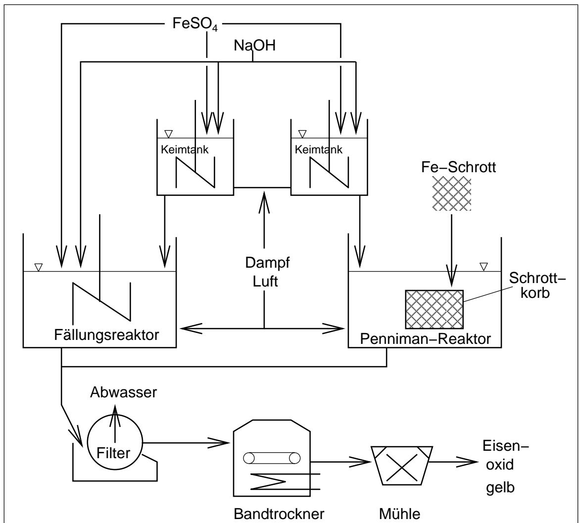
Produktion von Fe-Gelb durch Fällungs- (A) bzw. Penniman- (B) Prozess
