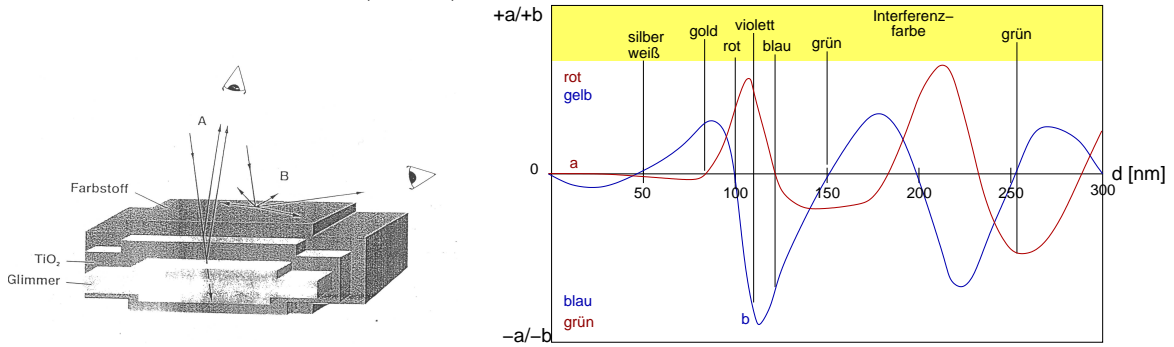
Aufbau (links) und Farben (rechts) von Glimmer/TiO 2 -Pigmenten
