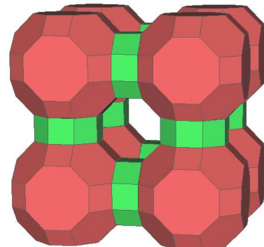
Rho
