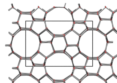
ZSM-5 (2. Ansicht)
