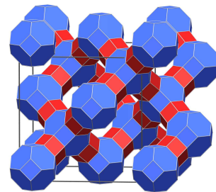
Faujasit
