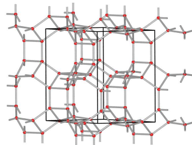
Phillipsit (lamellarer Z.)
