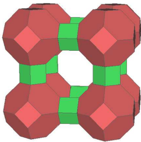
Linde A
