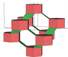
Chabazit (Polyeder)
