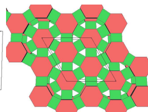
Chabazit
