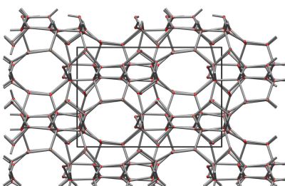
ZSM-5 (1. Ansicht)
