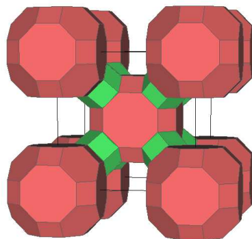
ZK-5
