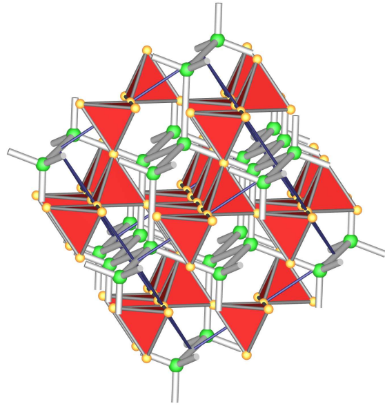
MgCu 2 : Gesamtstruktur
