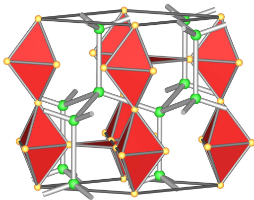
MgZn 2
