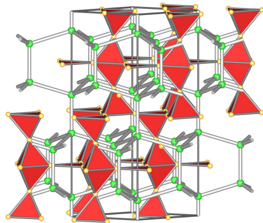
MgNi 2
