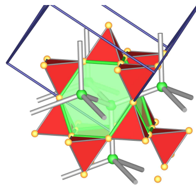
Mg-Umgebung: CN 12+4 (FK 16)
