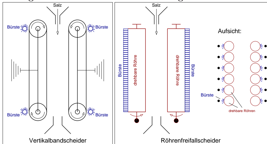
Bauarten von Elektroscheidern
