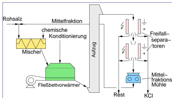
Fließschema zur NaCl/KCl-Trennung mittels Elektroscheidern
