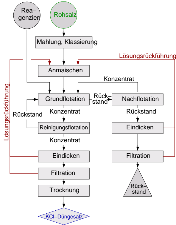
Prinzip der KCl/NaCl-Flotation
